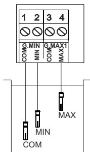
COMANDO ESTERNO 2 INGRESSI FUNZIONE RIEMPIMENTO
