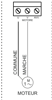
CONDENSATEUR SUR UNE POMPE
