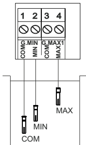
COMMANDE EXTÉRIEURE 2 ENTRÉES FONCTION REMPLISSAGE
